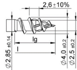
Filettatura a passo grosso II
