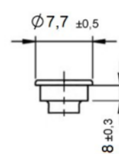
Testa con gradino
