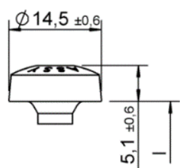
Testa cilindrica
