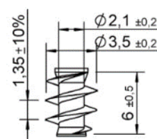
Filettatura sottotesta
