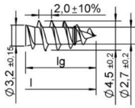
Filettatura semplice
