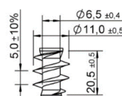
Filettatura sottotesta
