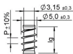
Filettatura sottotesta Lg2 < 4 \times d P = 2,2; 3,1; 4,4
