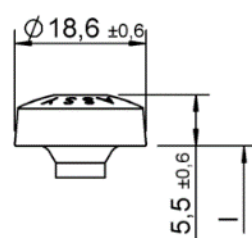
Testa cilindrica
