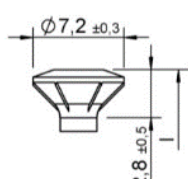
Testa FBS
