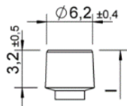
Testa cilindrica
