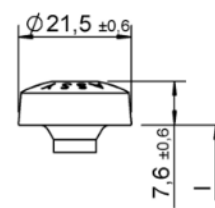
Testa cilindrica
