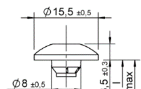
Testa per bandelle – con e senza bordi fresati o rinforzo del gambo
