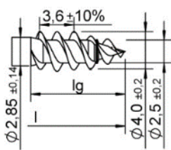
Doppia filettatura
