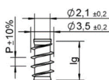
Filettatura sottotesta
