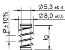
Filettatura sottotesta Lg2 < 4 \times d , P = 5,6
