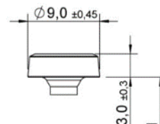
Testa Elmo
