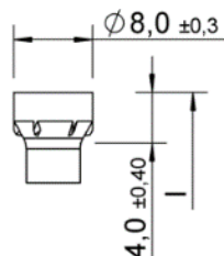
Testa cilindrica piccola – Versione con e senza bordi fresati
