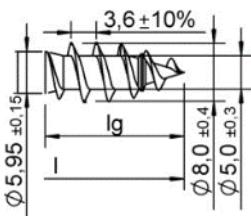
Filettatura semplice
