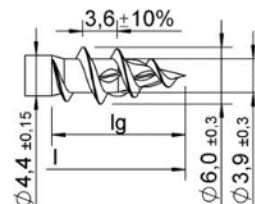
Filettatura a passo grosso II
