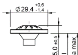
Testa a rondella larga/testa a bottone I
