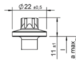
Testa rotonda esagonale esterna – con e senza colletto/rondella
