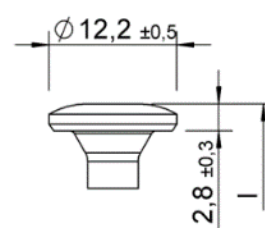
Testa cilindrica
