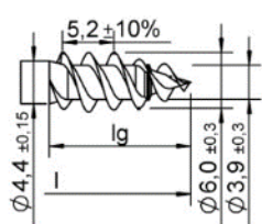
Doppia filettatura
