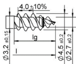
Doppia filettatura
