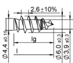
Filettatura semplice
