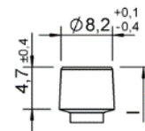
Testa cilindrica
