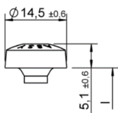
Testa cilindrica
