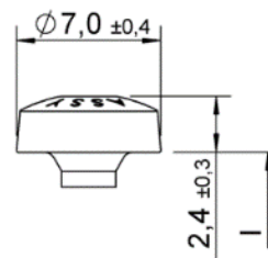
Testa cilindrica
