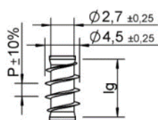
Filettatura sottotesta lg_2 < 4 \times d , P = 2,0; 2,8; 4,0
