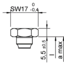
Testa combi – con e senza rinforzo del gambo/ Rondella
