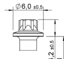
Testa rotonda esagonale esterna – con e senza rondella
