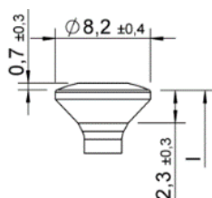
Testa per lamiera – con e senza bombatura
