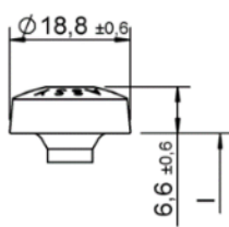
Testa cilindrica
