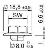
Testa esagonale – con e senza rinforzo del gambo/ rondella
