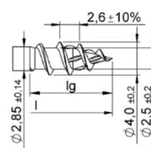
Filettatura a passo grosso II
