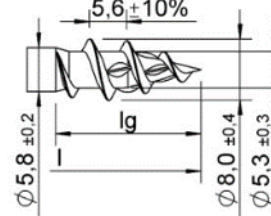
Filettatura a passo grosso II
