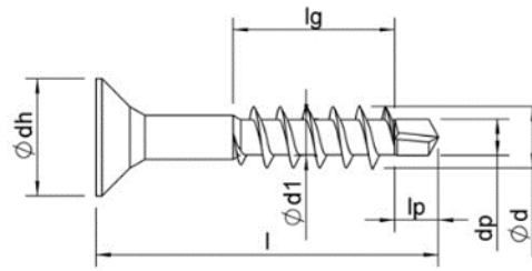
Filettatura parziale con punta perforante
