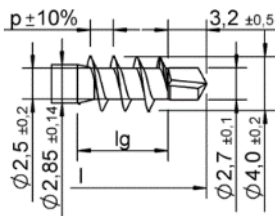
plus
