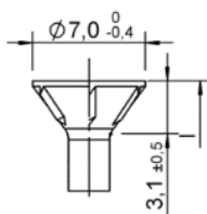
Testa svasata 75° – con e senza bombatura, con e senza incavature sottotesta
