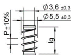
Filettatura sottotesta Lg2 < 4 \times d P = 1,8
