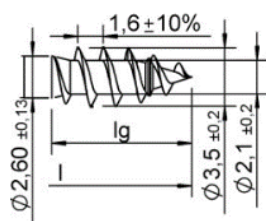
Filettatura semplice
