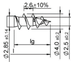
Filettatura a passo grosso I
