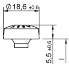
Testa cilindrica
