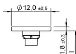
Testa a rondella larga/testa a bottone III - Versione con e senza bordi fresati
