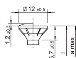
Testa svasata fresata – con e senza bombatura
