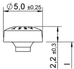
Testa cilindrica
