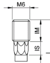
Testa per bandelle – con e senza bordi fresati o rinforzo del gambo
