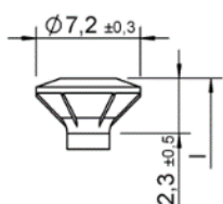
Testa FBS
