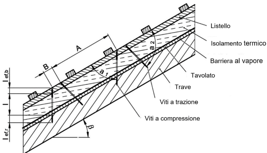
Figura A.7.4: Fissaggio dell'isolante a tetto sui puntoni - Rappresentazione schematica di viti disposte con inclinazione variabile
