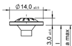
Testa a rondella larga/testa a bottone I
