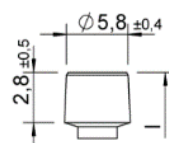
Testa cilindrica
