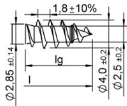
Filettatura semplice
