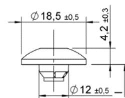
Testa per bandelle – con e senza bordi fresati o rinforzo del gambo
