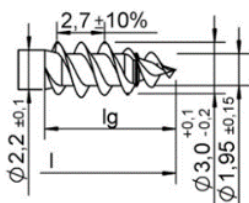
Filettatura semplice
