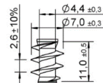
Filettatura sottotesta
