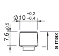
Testa cilindrica
