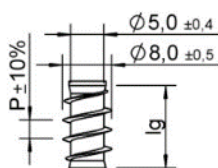
Filettatura sottotesta Lg2 < 4 \times d , P = 3,6
