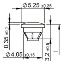
Top head – con e senza bombatura
