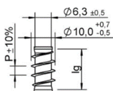
Filettatura sottotesta
