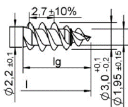
Doppia filettatura
