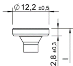
Testa piatta
