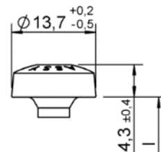
Testa cilindrica
