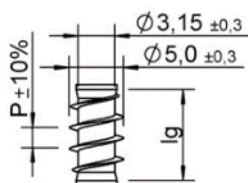
Filettatura sottotesta Lg2 < 4 \times d , P = 4,6
