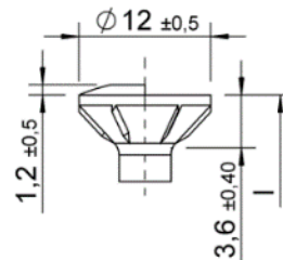
Testa svasata fresata – con e senza bombatura
