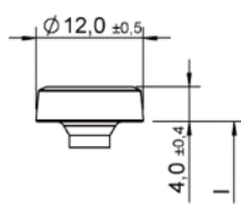
Testa Elmo
