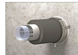
Fig. 3: Tubo multistrato
