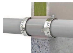
Fig. 1: Tubo lineare
