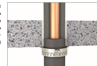
Fig. 6: Tubo metallico con collare (nastro intumescente + nastro metallico)
