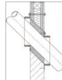
Fig. 4: Tubo metallico con nastro intumescente all'interno della parete (senza uso del nastro metallico)
