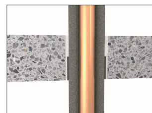
Fig. 5: Tubo metallico con due nastri intumescenti affiancati all'interno del solaio (senza uso del nastro metallico)
