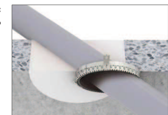
Fig. 2: Tubo inclinato
