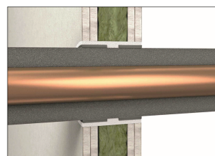
Fig. 4: Tubo metallico con nastro intumescente all'interno della parete (senza uso del nastro metallico)
